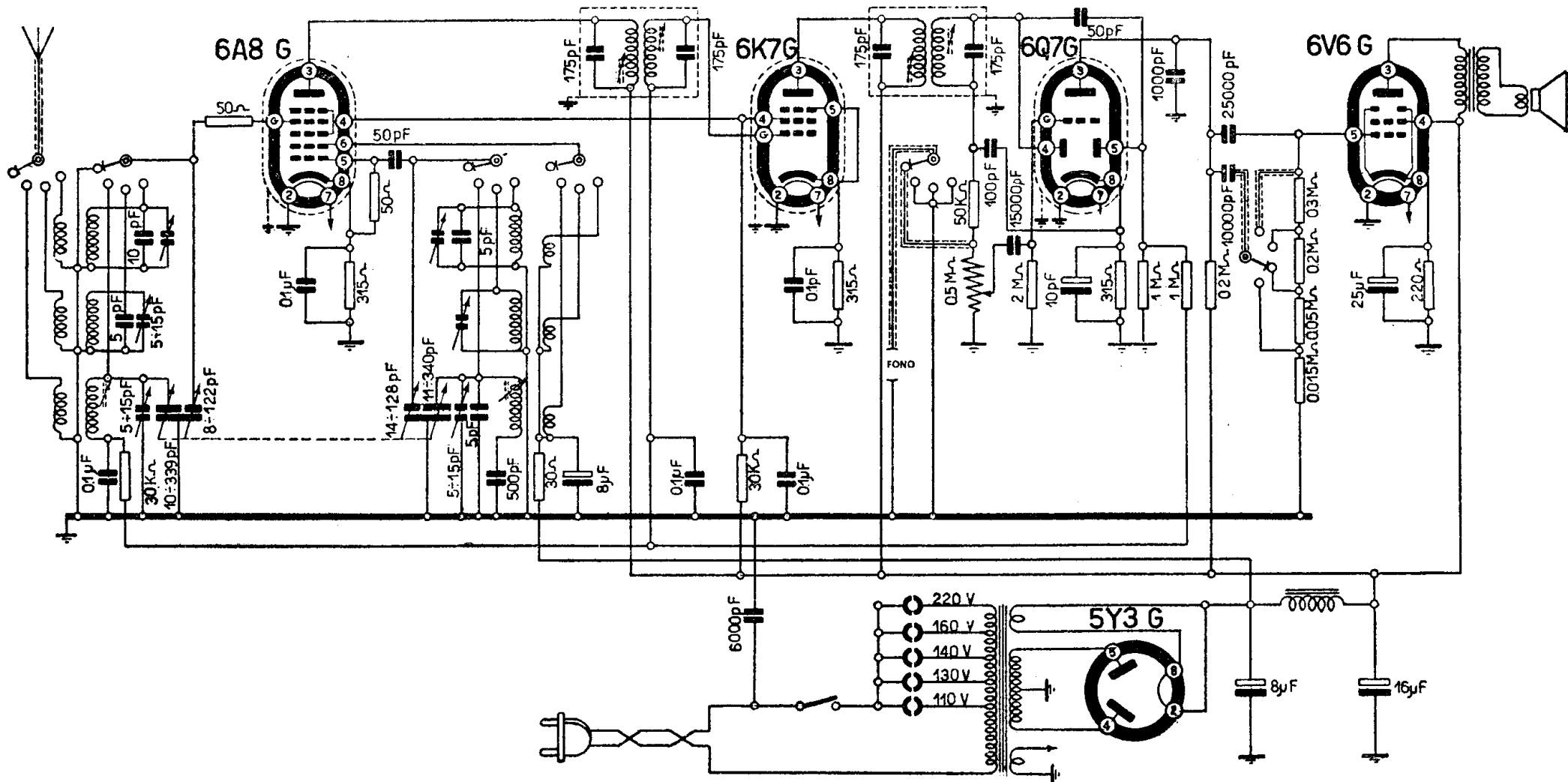
DUCATI - Mod. RR 3411.1 - Apparecchio da tavolo. Gamme: da 190 a 570 m, da 28 a 50 m e da 16 a 28 m. Media frequenza: 468 kc/s. Sensibilità: 40 µV. Potenza: 4 watt. Produzione 1946 (v. tabella a parte).
